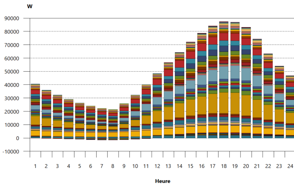
Évolution horaire de la charge maximale simultanée de refroidissement (21 Août)
